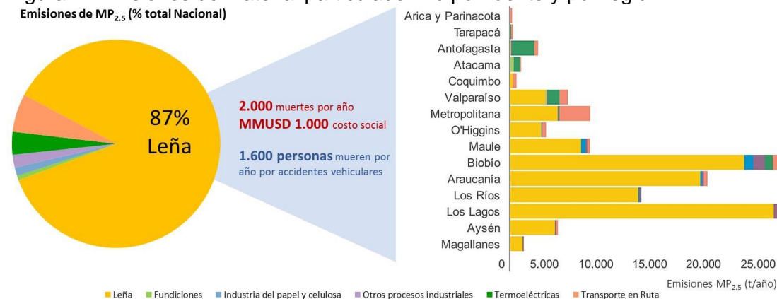
Figura 2: Emisiones de material particulado fino por fuente y por región
